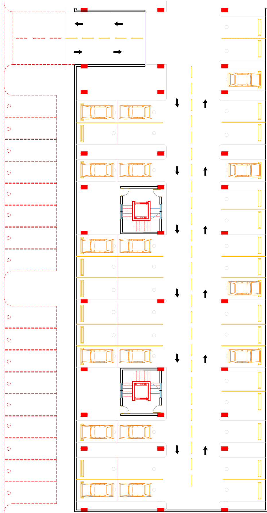
2 PLANTA ARQUITECTONICA BLOQUE "A" PARQUEOS ESC: 1/75 A.1.1 ORGANIZACION PARQUEOS
